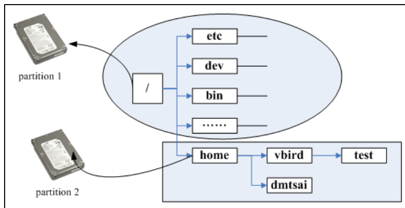
图2.2.10、目录树与分区之间的相关性
