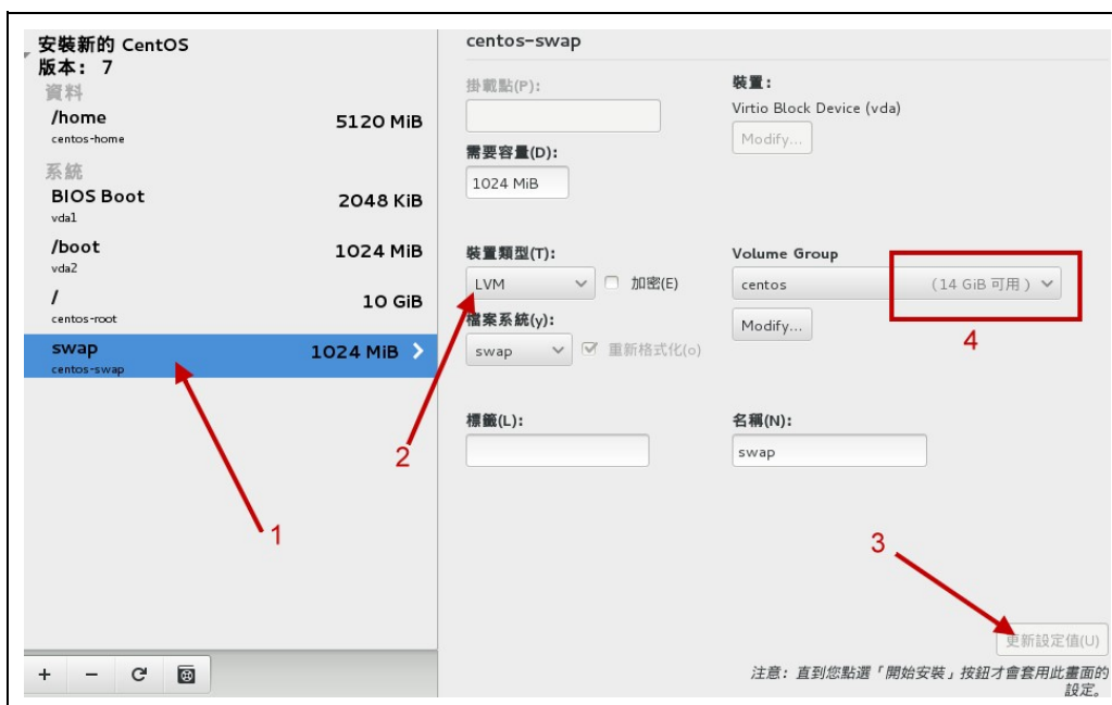
图3.2.30、调整 swap 也使用 LVM 设备
