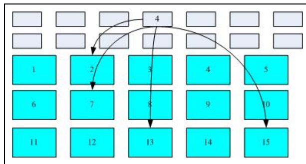
图7.1.1、inode/block 数据存取示意图
