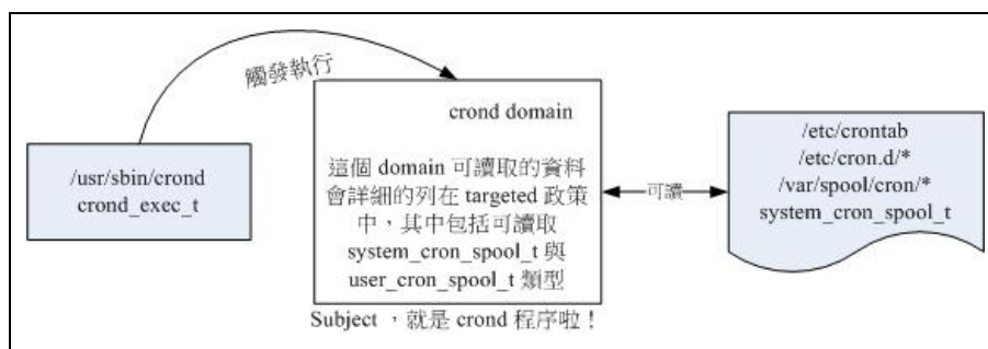
图16.5.3、主体程序取得的 domain 与目标文件资源的 type 相互关系以 crond 为例
