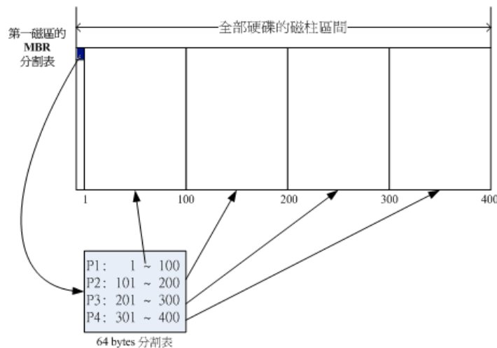
图2.2.2、磁盘分区表的作用示意图
