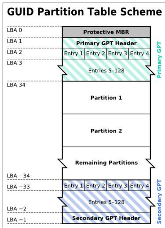
图2.2.7、GPT分区表的结构示意图
