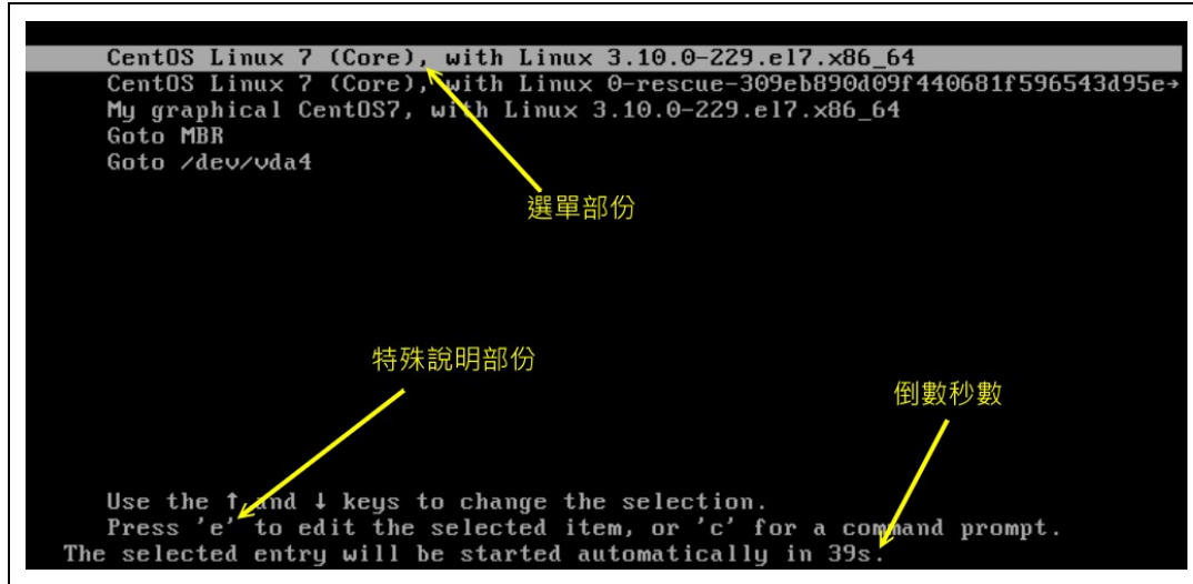
图19.3.1、grub2 开机画面示意图
