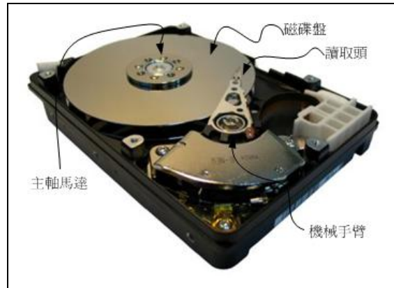
图0.2.4、硬盘物理构造（图片取自维基百科）
