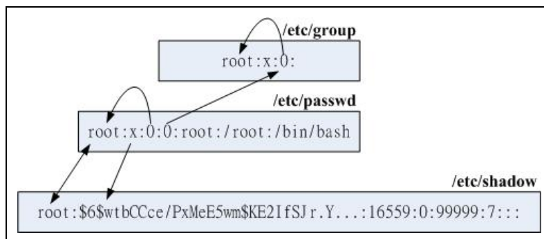
图13.1.1、帐号相关文件之间的 UID/GID 与密码相关性示意图
