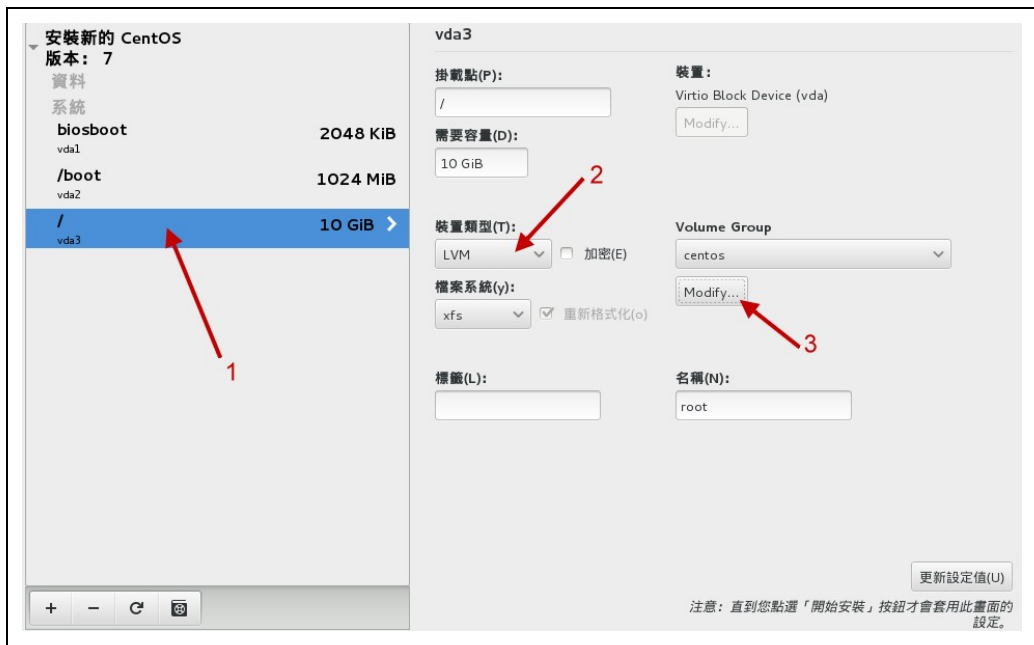
图3.2.25、将设备类型改为 LVM 的管理机制
