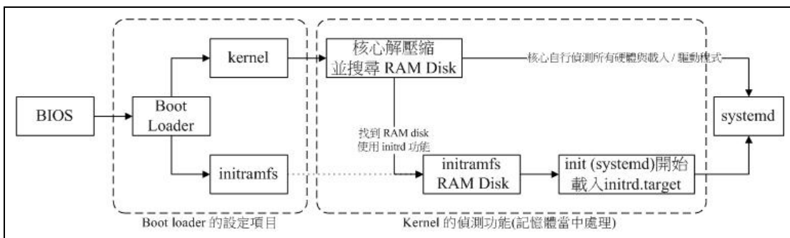
图19.1.3、BIOS 与 boot loader 及核心载入流程示意图
