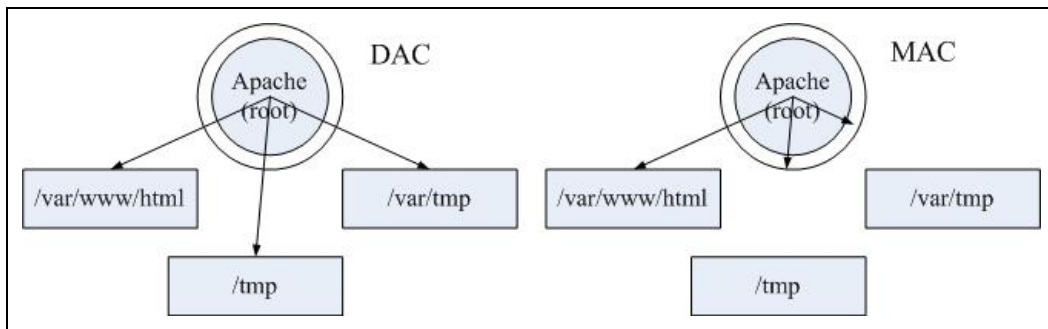
图16.5.1、使用 DAC/MAC 产生的不同结果，以 Apache 为例说明
