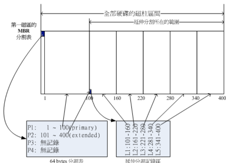
图2.2.3、磁盘分区表的作用示意图
