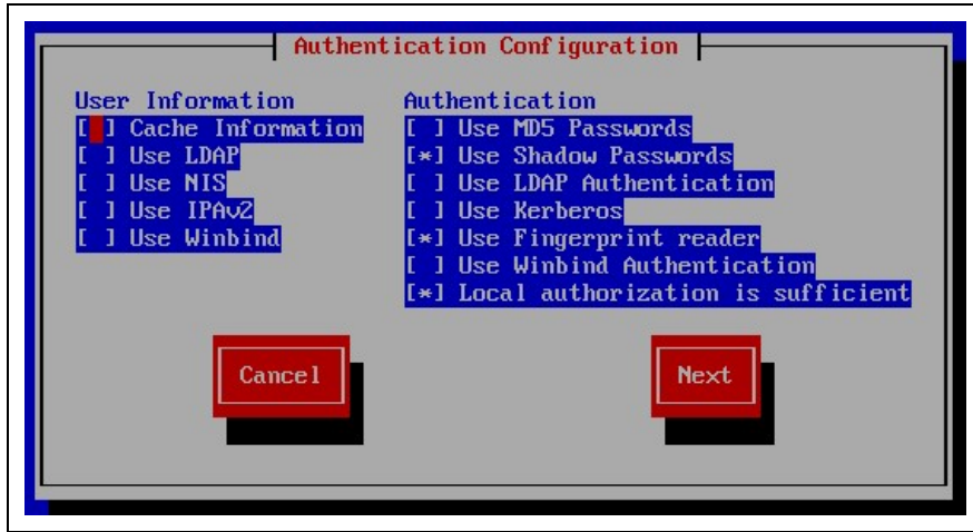
图13.2.1、使用外部身份验证服务器的方式
