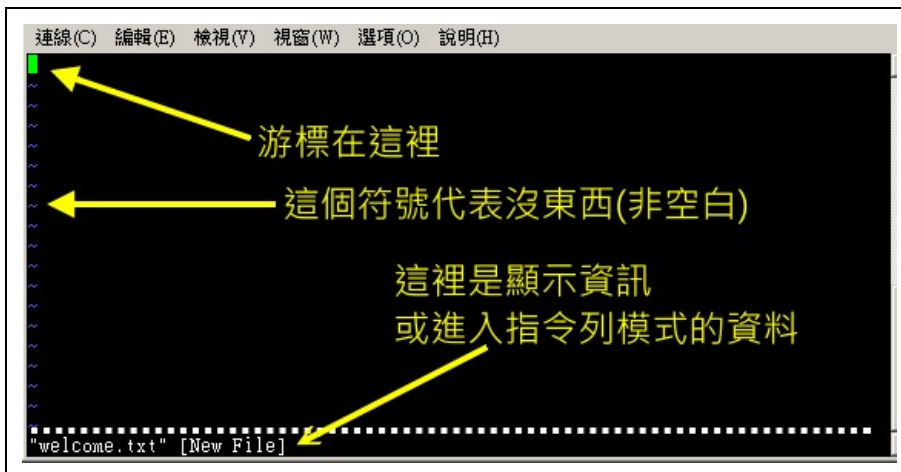
图9.2.2、用 vi 打开一个新文件
