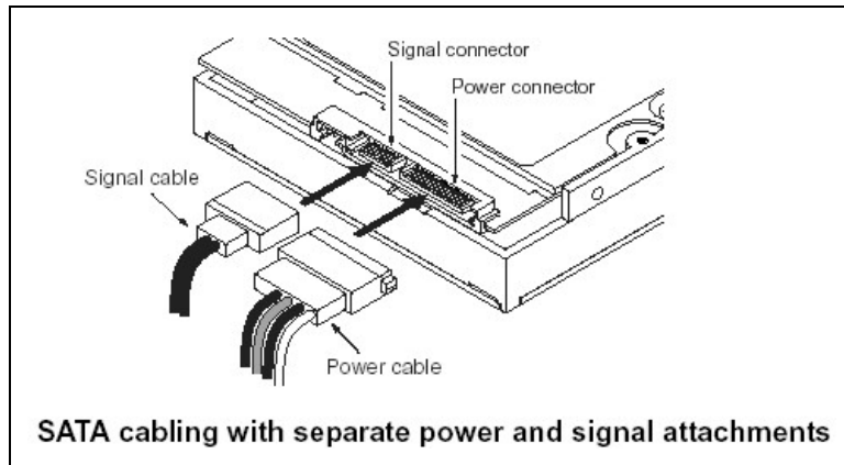
图0.2.6、SATA 接口的排线（图示取自 Seagate 网站）
