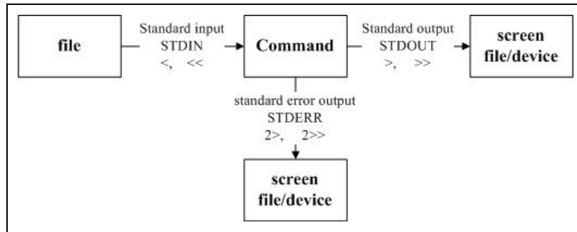
图10.5.1、指令执行过程的数据传输情况
