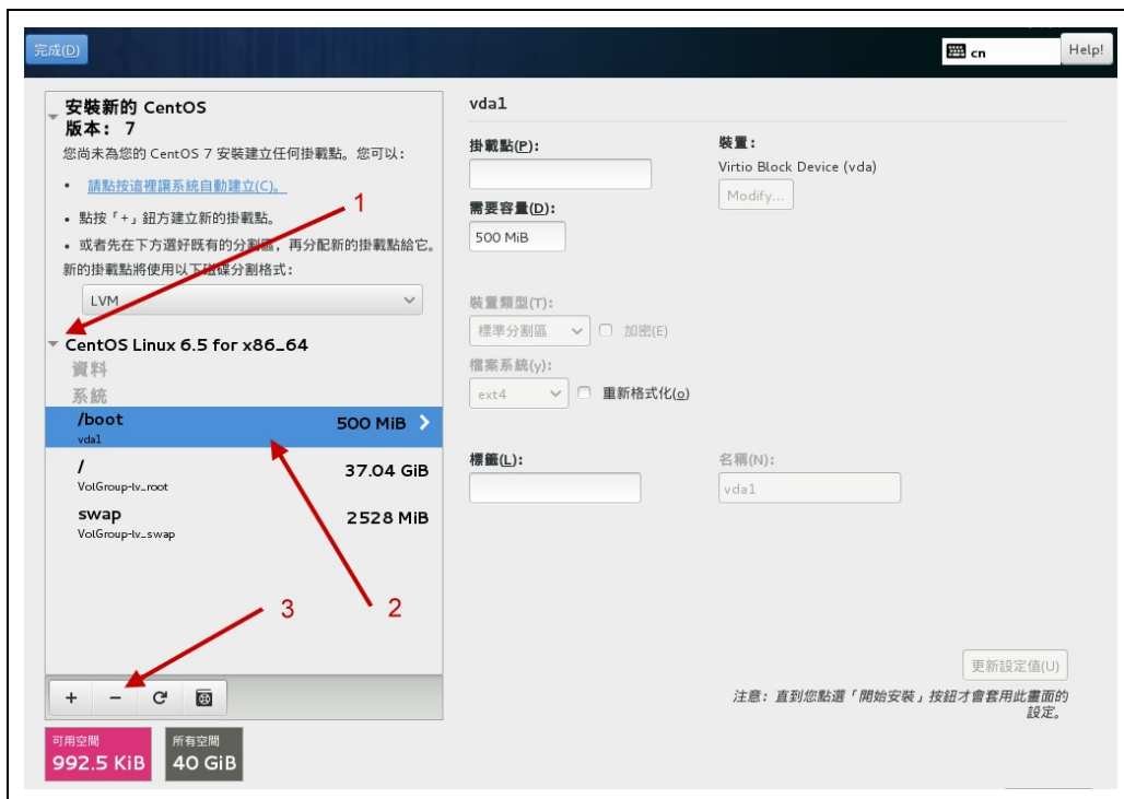
图3.2.19、删除已经存在系统当中的分区
