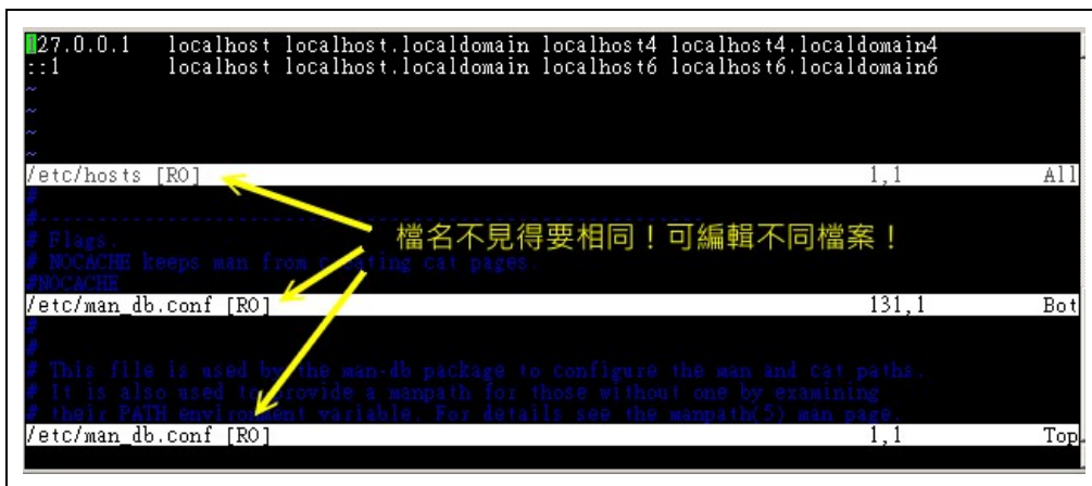
图9.3.8、vim 的窗口分区示意图
