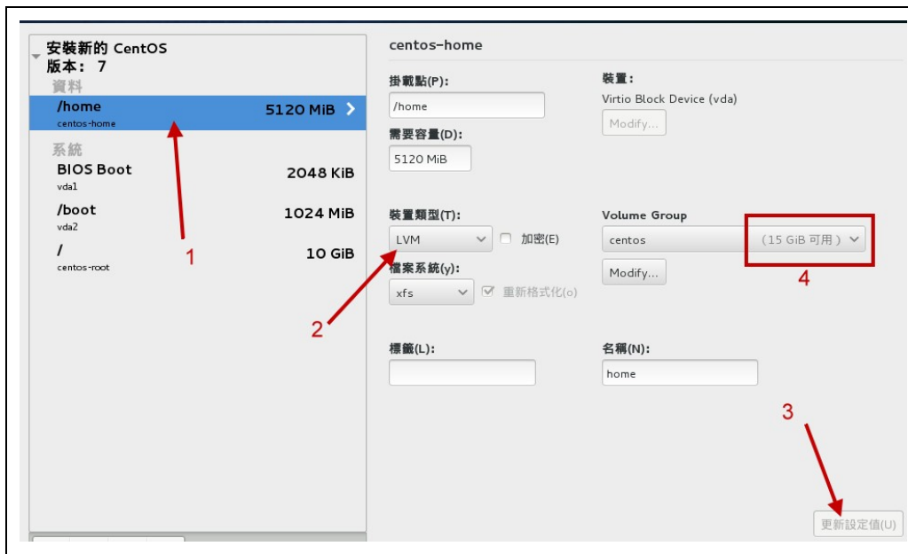
图3.2.28、调整 /home 也使用 LVM 设备
