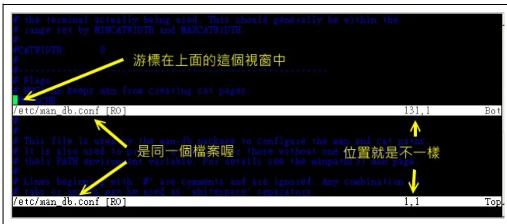
图9.3.7、vim 的窗口分区示意图
