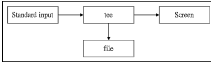
图10.6.2、tee 的工作流程示意图
