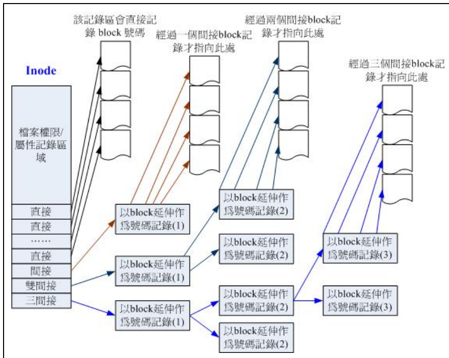
图7.1.4、inode 结构示意图
