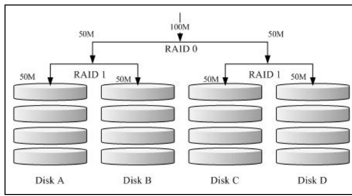
图14.2.3、RAID-1+0 的磁盘写入示意图
