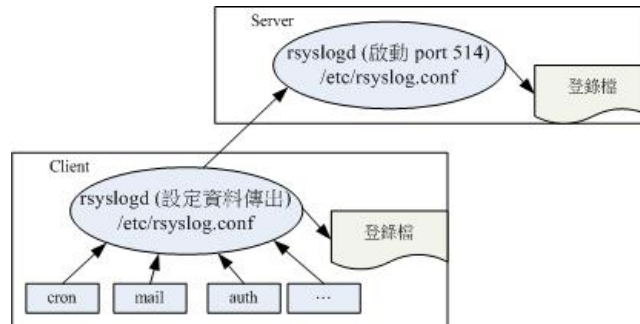
图18.2.2、登录文件服务器的架构
