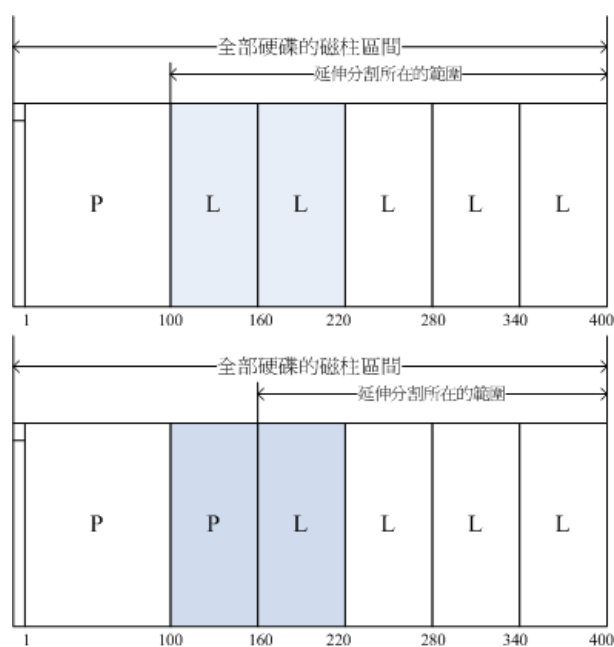
图2.2.4、磁盘空间整合示意图
