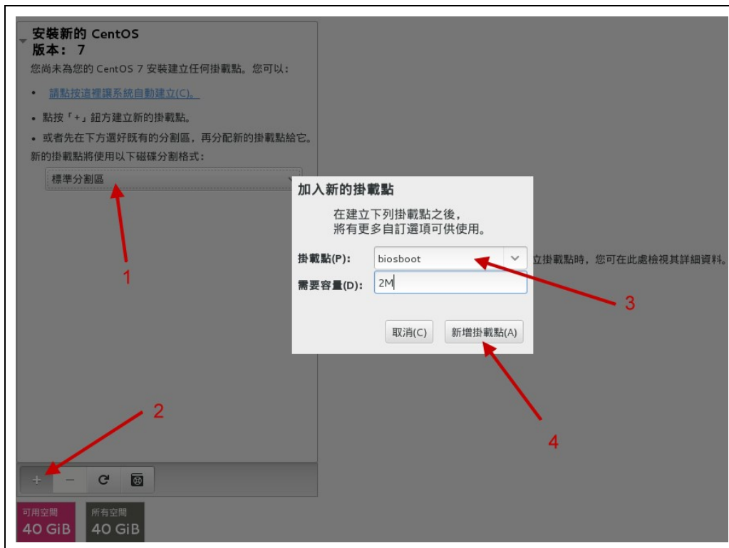
图3.2.21、创建 BIOS boot 分区的示意图
