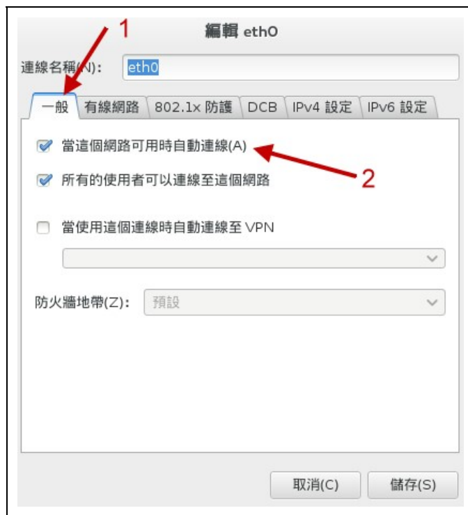
图3.2.35、设置开机自动启动网络
