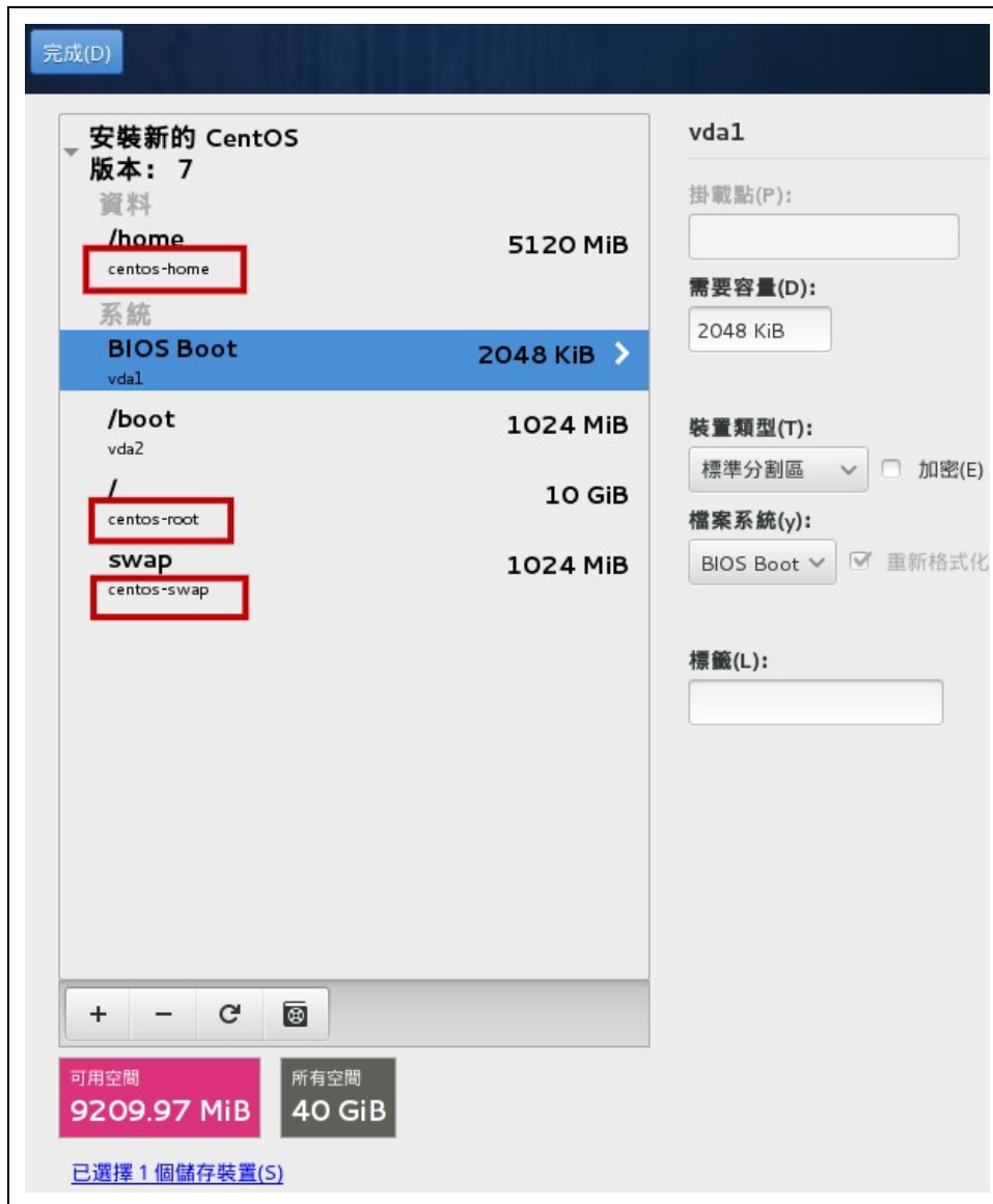
图3.2.31、完成分区之后的示意图
