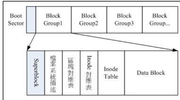
图7.1.3、ext2文件系统示意图 [1]
