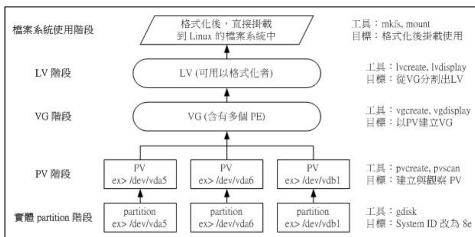
图14.3.2、LVM 各元件的实现流程图示
