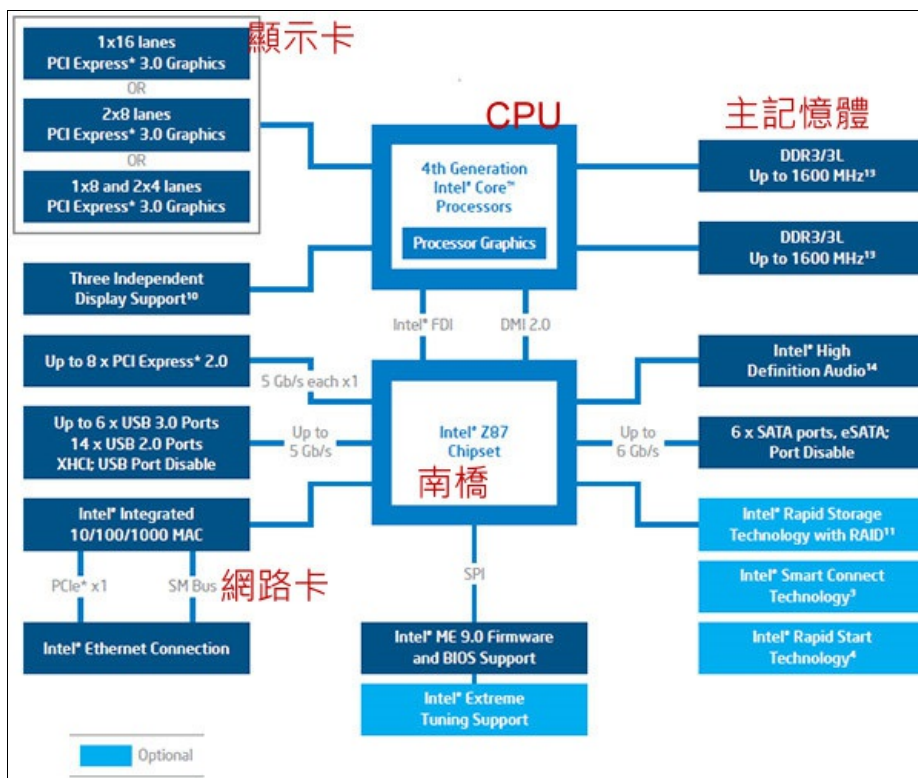
图 0.2.1、Intel 芯片架构
