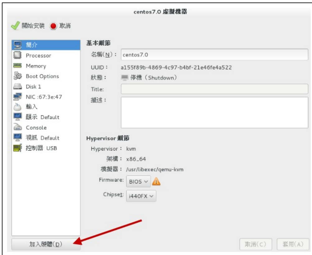
图3.2.5、设置完成的示意图
