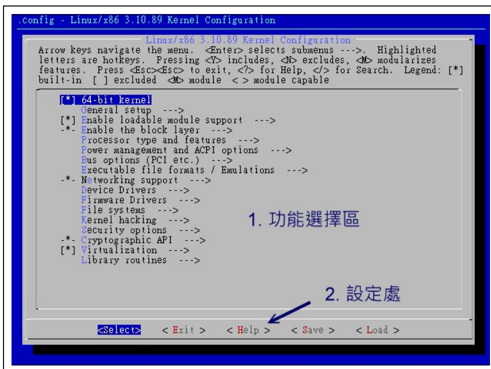
图24.2.1、make menuconfig 核心功能挑选菜单示意图
