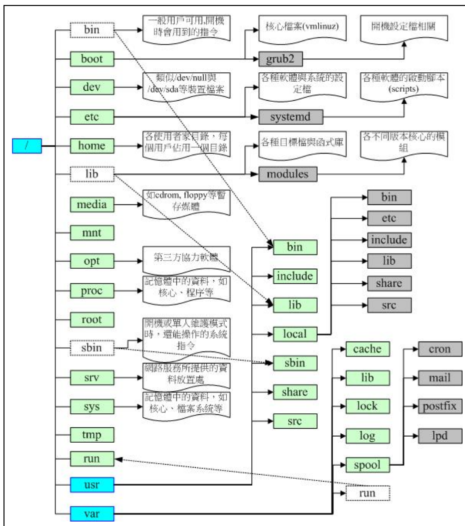
图5.3.1、目录树架构示意图
