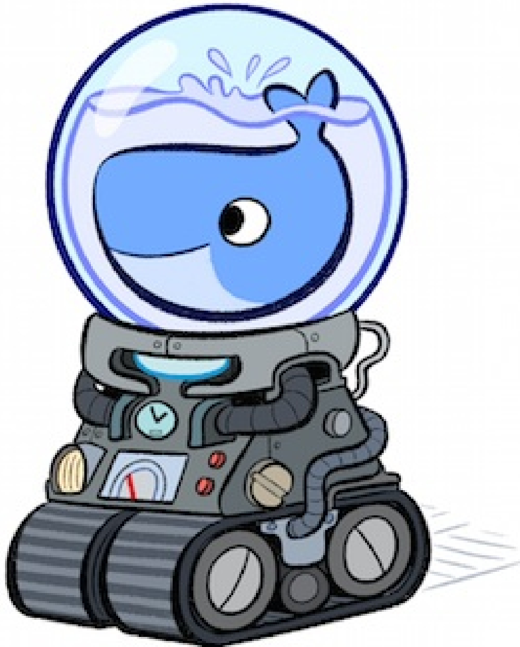
图 1.17.1.1 - Docker Machine
